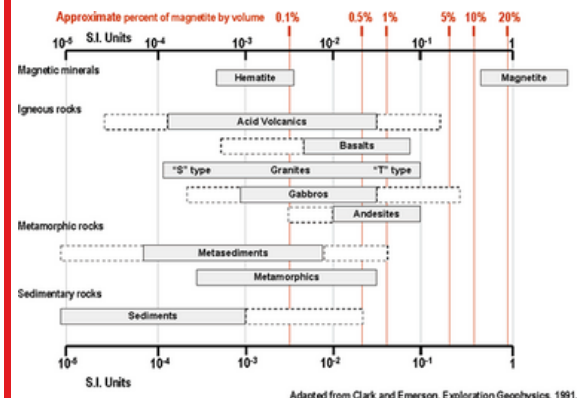
Susceptibilidad magnética de tipos de rocas comunes.
